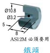
MB12M
