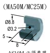
鐵頭
