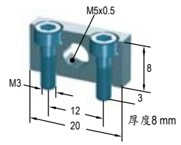
固定架
