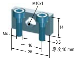
固定架
