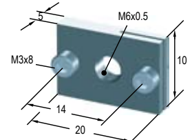
夾溝槽法蘭
