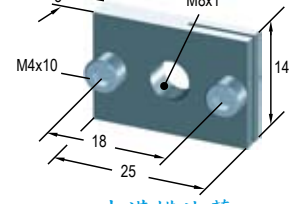
夾溝槽法蘭
