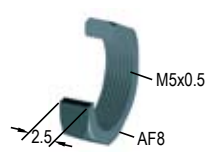
螺母
