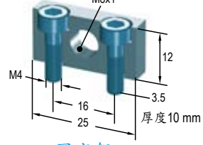
固定架
